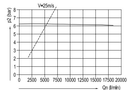
Curva de caudal del filtro QBS9
