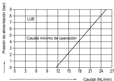
Curva de goteo del lubricador QBS4
