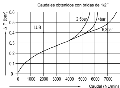
Curva de caudal del lubricador QBS4
